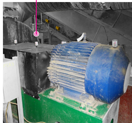
Een FGR ventilator gesmeerd door een simalube 60 ml smeerpatroon.
